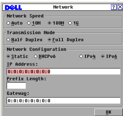
Рис. 3-10. Диалоговое окно «Network» (режим IPv6)
