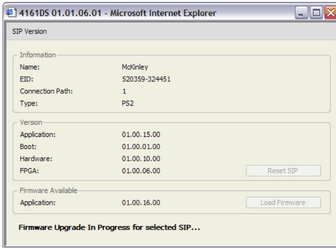
Рис. 6-16. Окно «SIP Version»
