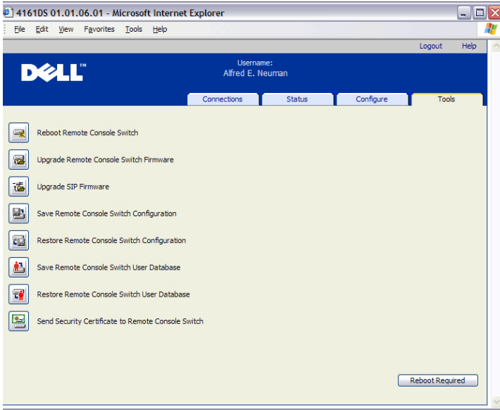
Рис. 8-3. Встроенный веб-интерфейс — отправка сертификата безопасности
