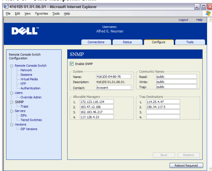
Рис. 6-5. Окно настройки SNMP
