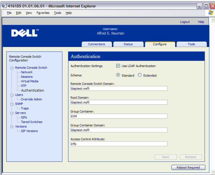
Рис. 8-2. Встроенный веб-интерфейс — панель аутентификации для локального входа/LDAP и параметры
