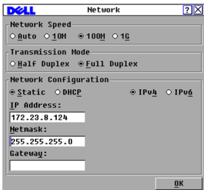
Рис. 3-9. Диалоговое окно «Network» (режим IPv4)
