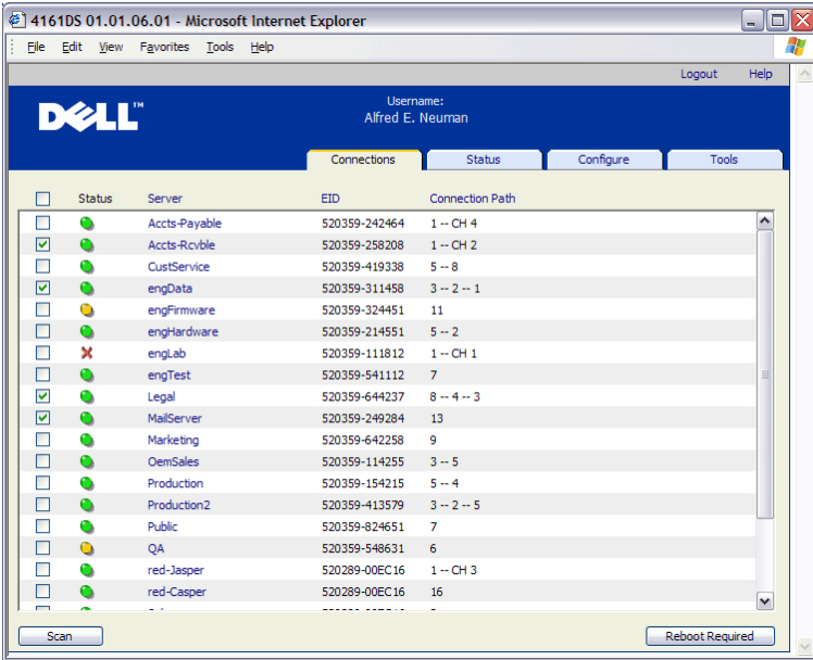
Рис. 4-10. Встроенный веб-интерфейс — сканирование серверов
