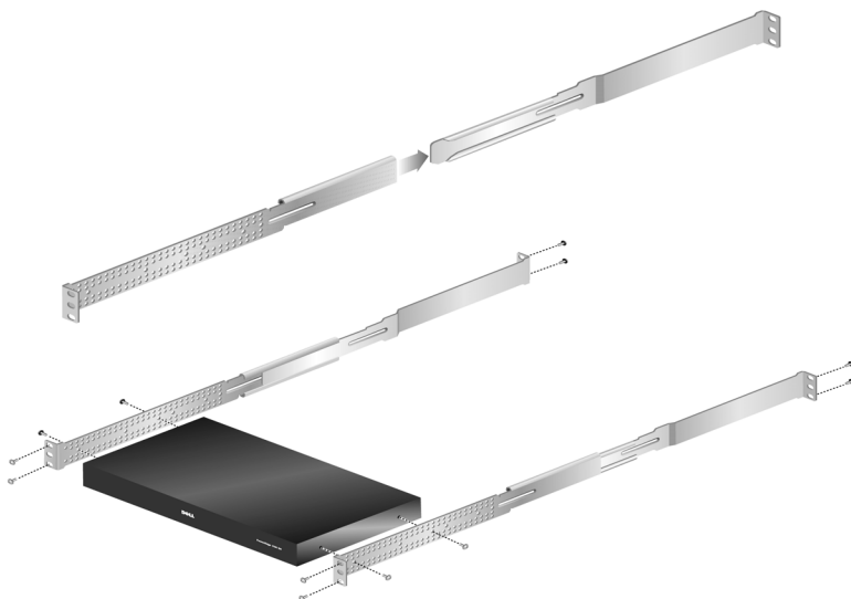
Рис. 2-2. Установка монтажного кронштейна удаленного консольного коммутатора 2161DS-2/4161DS 1U
