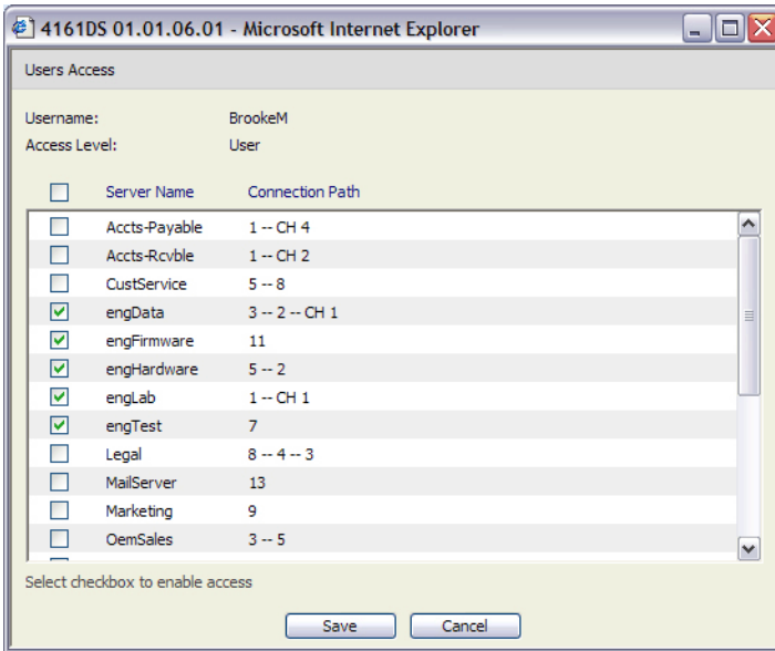
Рис. 6-4. Окно прав доступа пользователя
