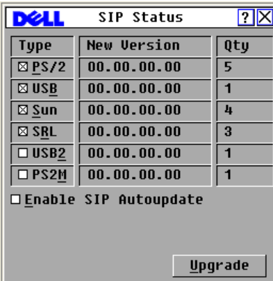
Рис. Г-2. Диалоговое окно «SIP Status»
