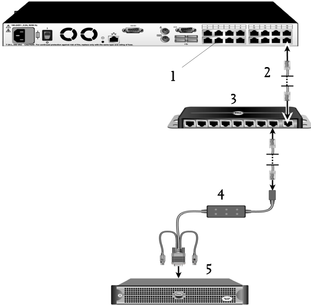
Рис. 2-14. Конфигурация удаленного консольного коммутатора с модулем PEM
