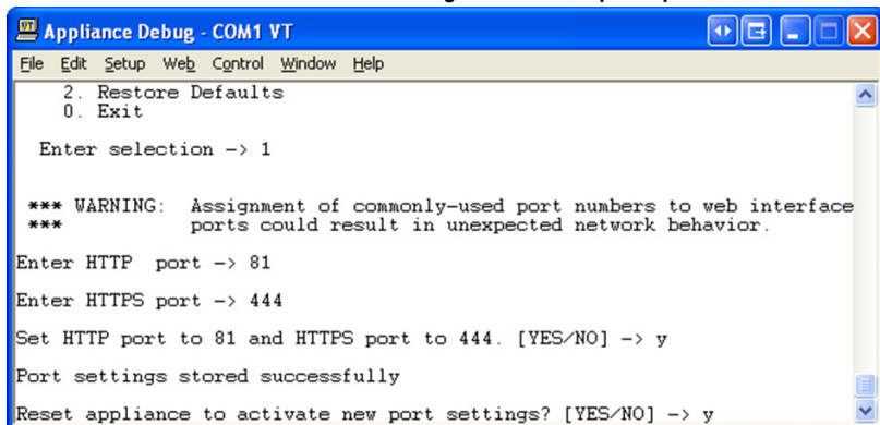
Рис. 2-8. Меню «Web Interface Port Configuration» — параметр «Set Ports»
