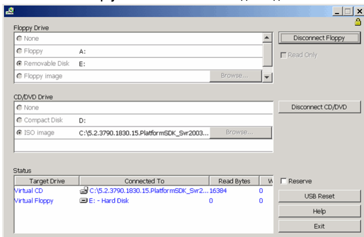
Рис. 5-5. Клиент виртуального носителя Dell — два подключения
