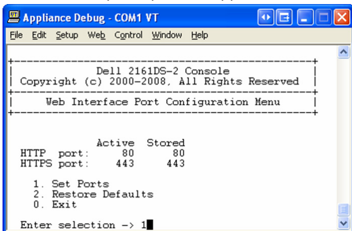
Рис. 2-7. Меню настройки портов веб-интерфейса
