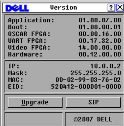
Рис. 3-11. Диалоговое окно «Version»
