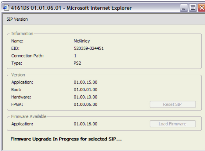
Рис. 6-13. Окно «SIP Version»
