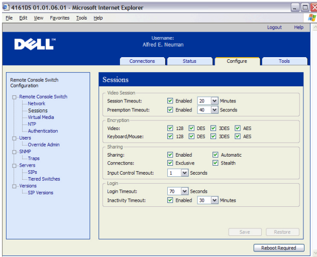
Рис. 8-5. Встроенный веб-интерфейс — меню «Login Timeout»
